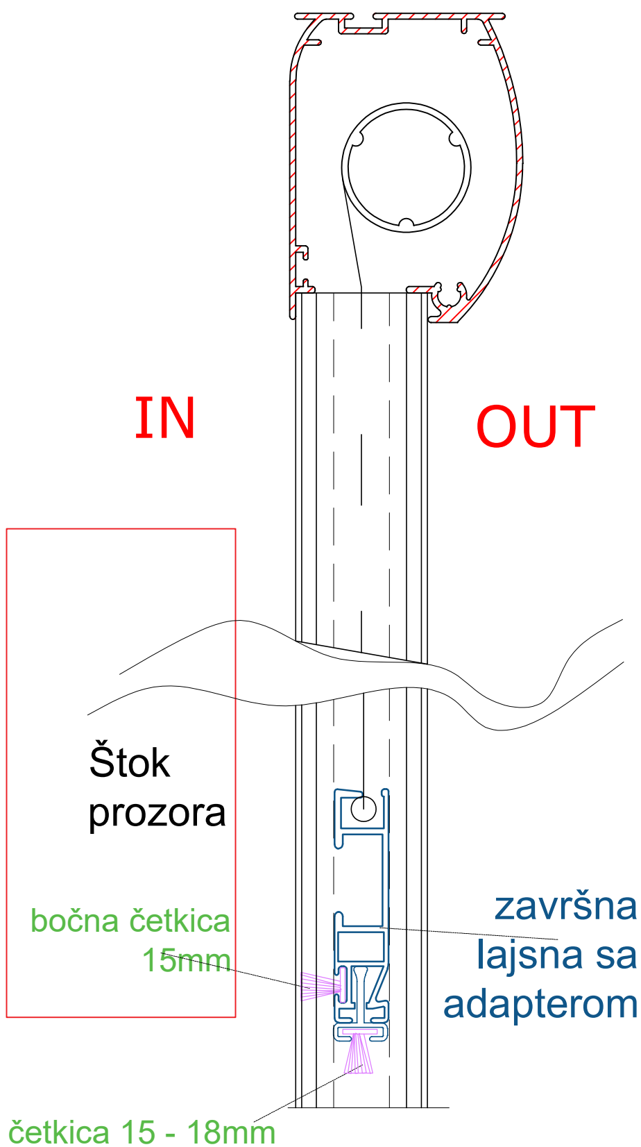
Vertikalni presek
