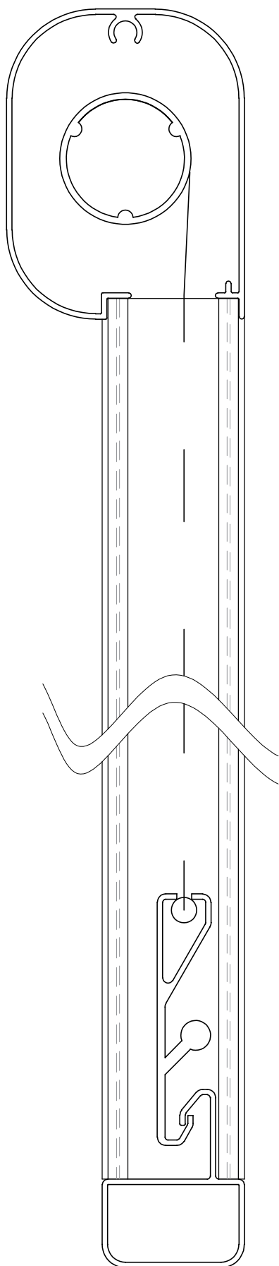
Vertikalni presek
